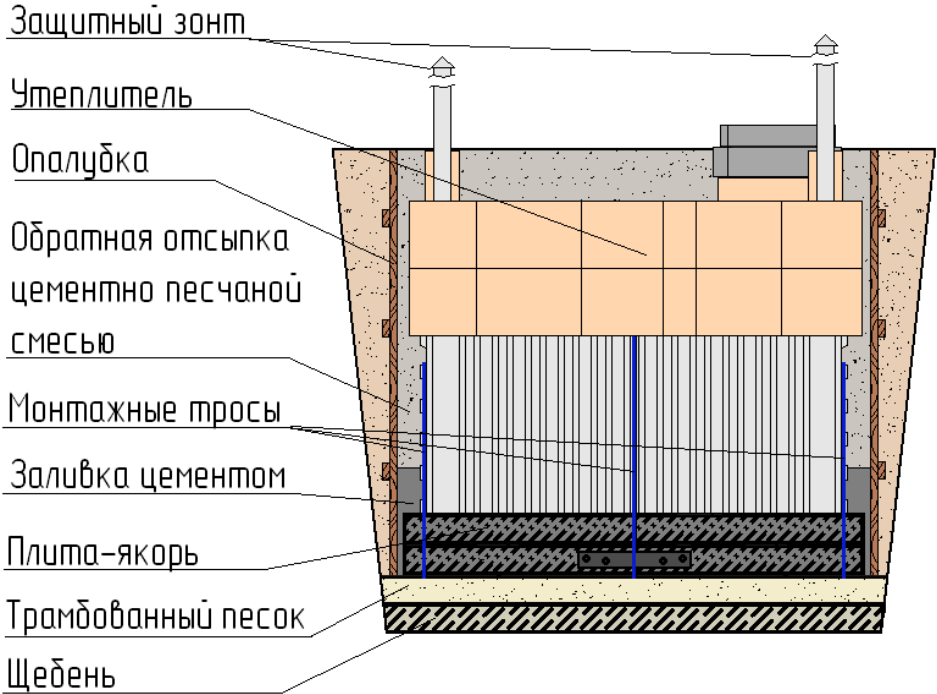
Схема монтажа погреба Т3000 с нижним якорением (Схема подходит для погребов моделей Т2500, Т3000, Т3500)
