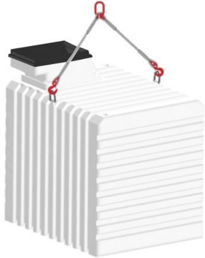
Рисунок 4. Крепление стропой СТП-1
