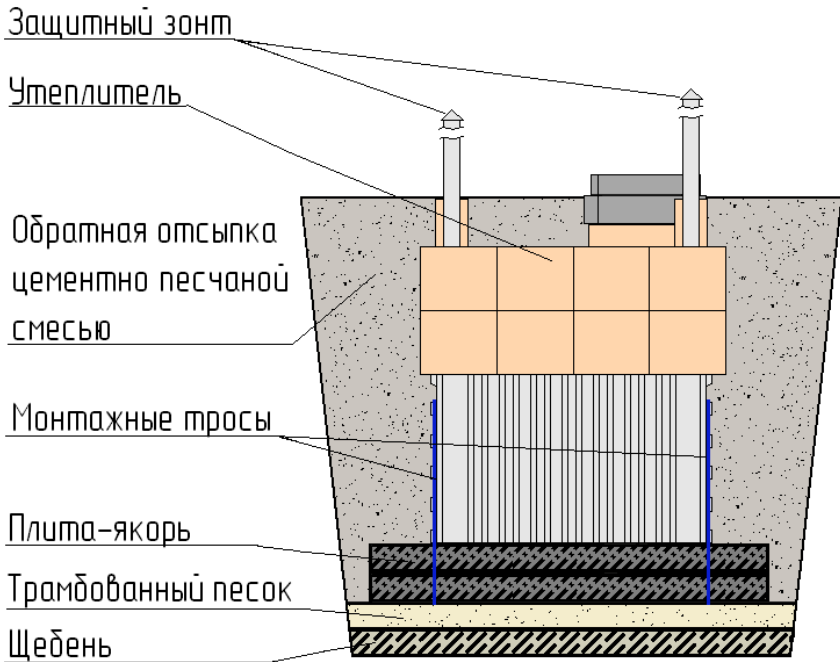
Схема монтажа погреба Т1900 с нижним якорением (Схема подходит для погребов моделей Т1900, Т2500)
