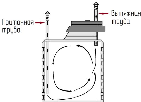
Рисунок 7. Схема циркуляции воздуха в приточно-вытяжной вентиляции.
