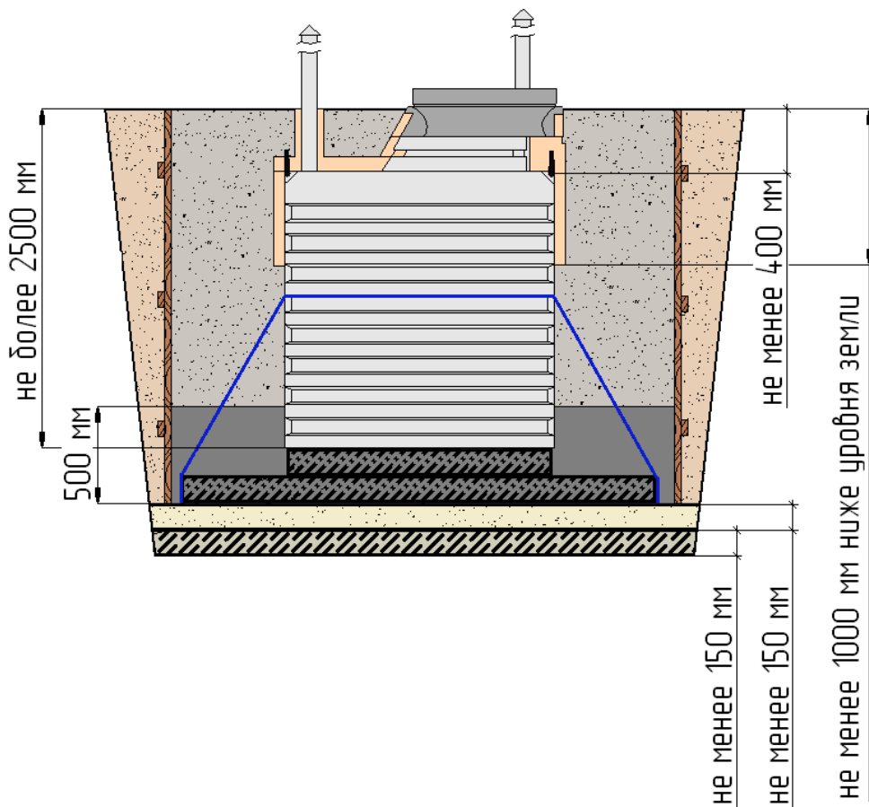
Схема монтажа погребов Т3000 с нижним якорением (Схема подходит для погребов моделей Т2500, Т3000, Т3500)
